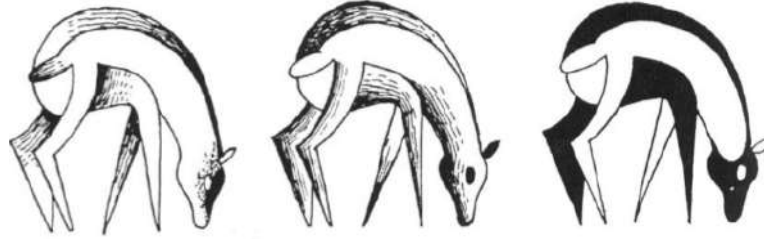
Şekil 13: Sadeleştirme Tekniği
